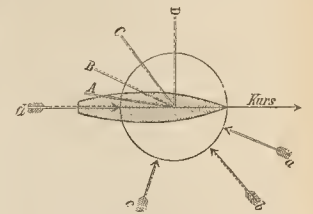
Fig. 5. Distintas posiciones de la vela mayor según la dirección del viento
